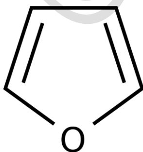
(Furan)
