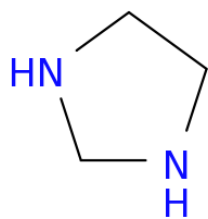
(Imidazolidine)
