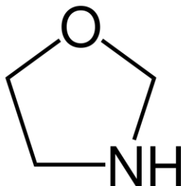
(Oxazolidine)
