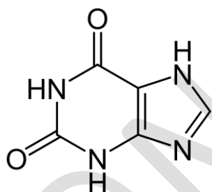
(Xanthine)
