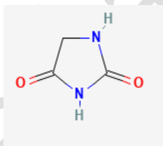
(Hydantoin)
