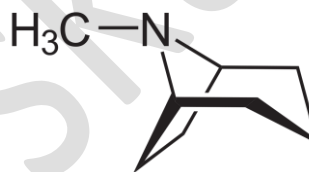
(Tropane)
